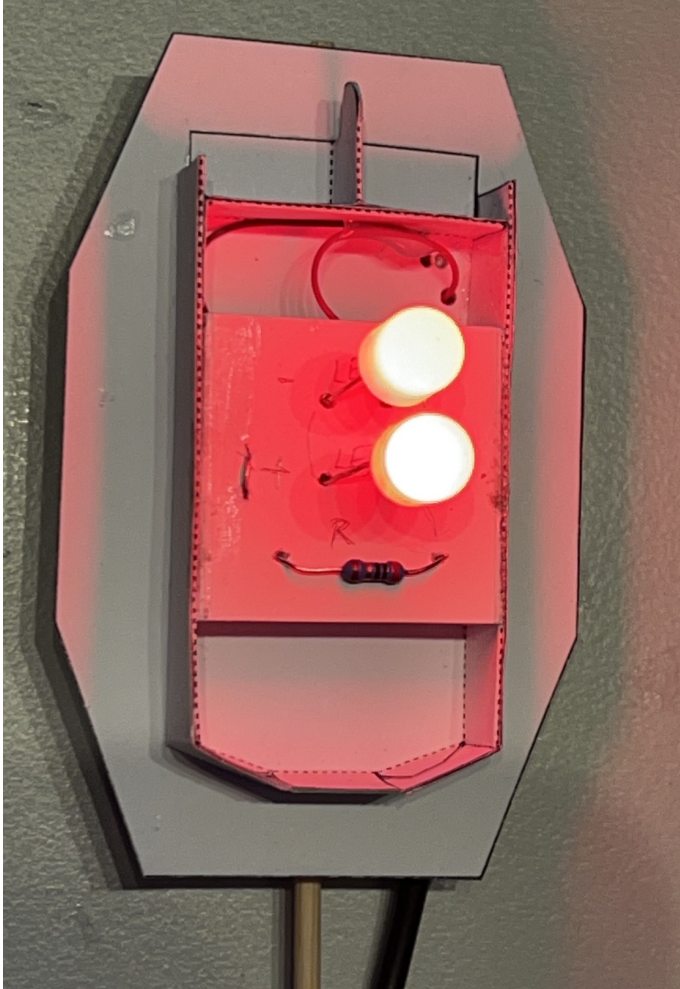
Bild: Die Halterung wurde mit zwei 360 Grad LEDs bestückt.
