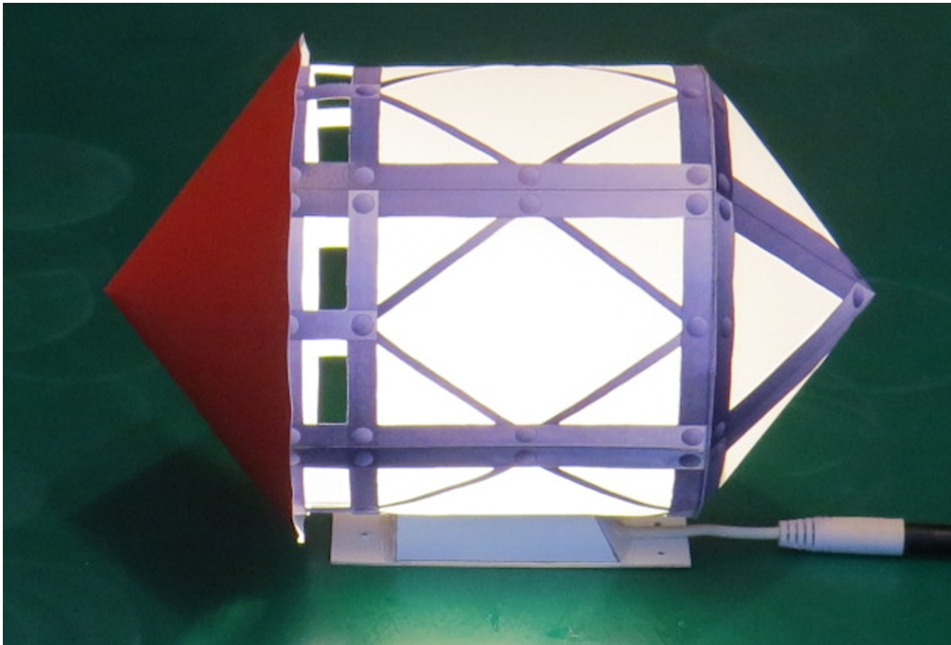
Die Laterne wurde auf die Fassung gesetzt. Zum Betrieb wurde eine LED-Leuchtmittel mit G4-Anschluß verwendet.
