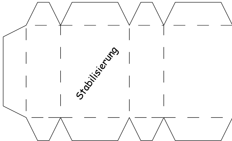
Darstellung: Lage der Stabilisierungen im LKW
